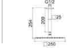
GRIFERÍA TERMOSTÁTICA
