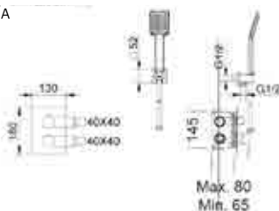
GRIFERÍA
